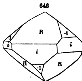
C. Blomidon.
